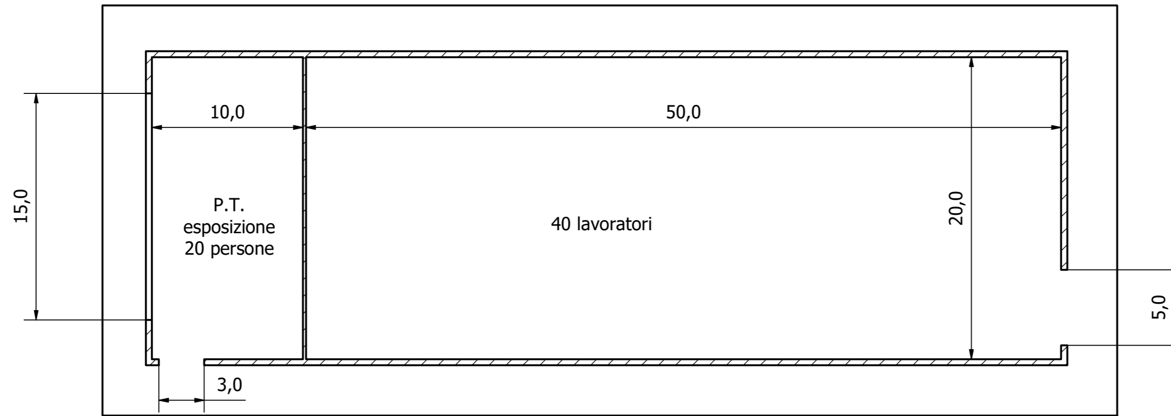
A-A ( 1 : 250 )
